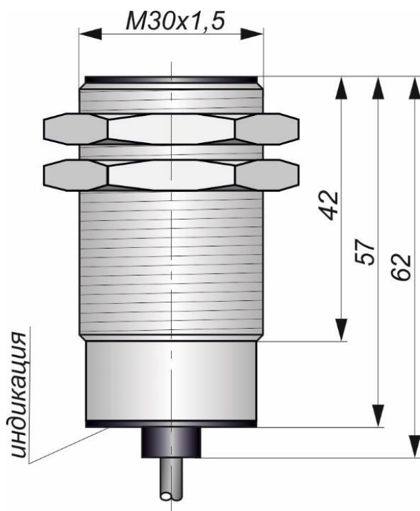
Габаритный чертеж
